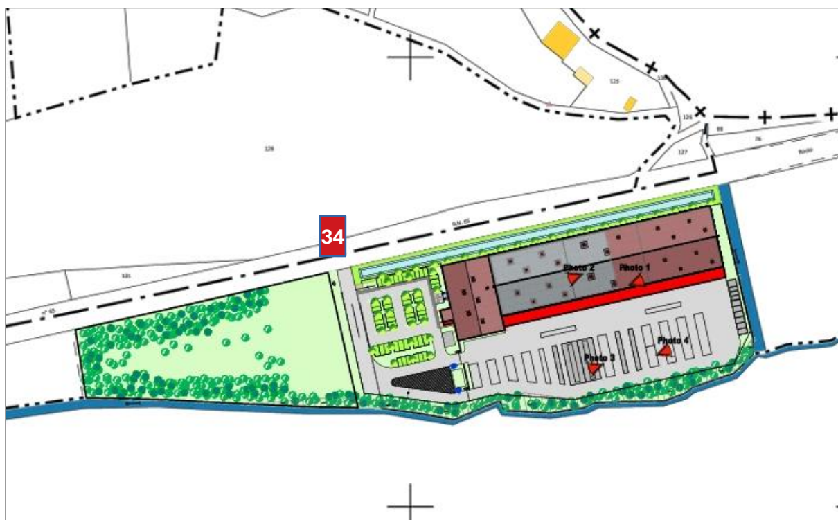
Plan de masse du projet de construction – PC 089 024 25 00013
